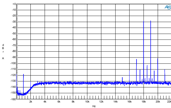
CCIF FFT, Channel 1, f_1=18 khz, f_2=19 khz R_L=4 Ohm, P_0=10 W.
