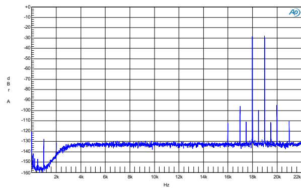
CCIF FFT, Channel 2/3, f_1=18 khz, f_2=19 khz R_L=4 Ohm, P_0=10 W.
