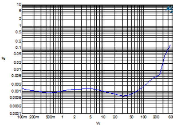
CCIF vs power R_L=4 ohm, SE, f_1=18 kHz, f_2=19 kHz
