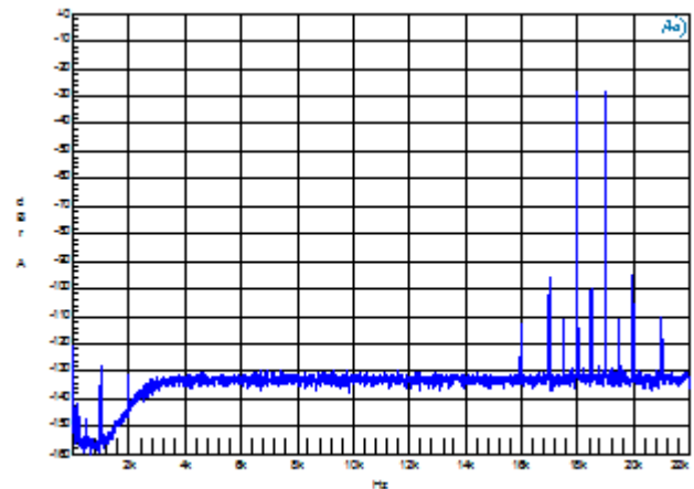
CCIF FFT, SE, f_1=18 kHz, f_2=19 kHz, R_L=40 hm, P_O=10 W.
